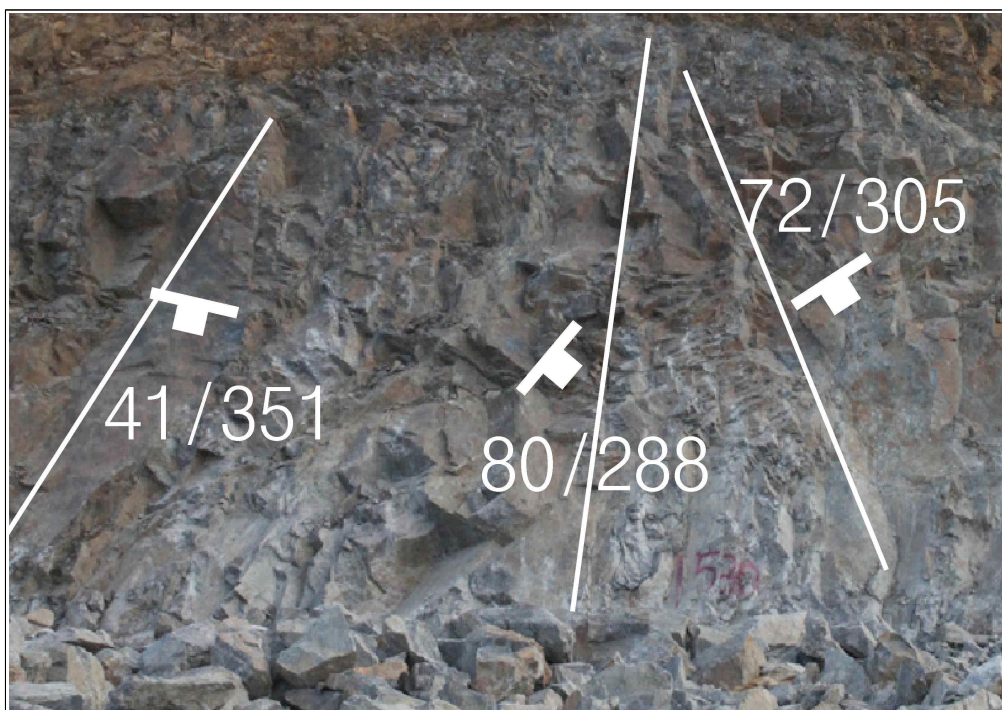
【그림 13】 A 영역에 발달한 불연속면
