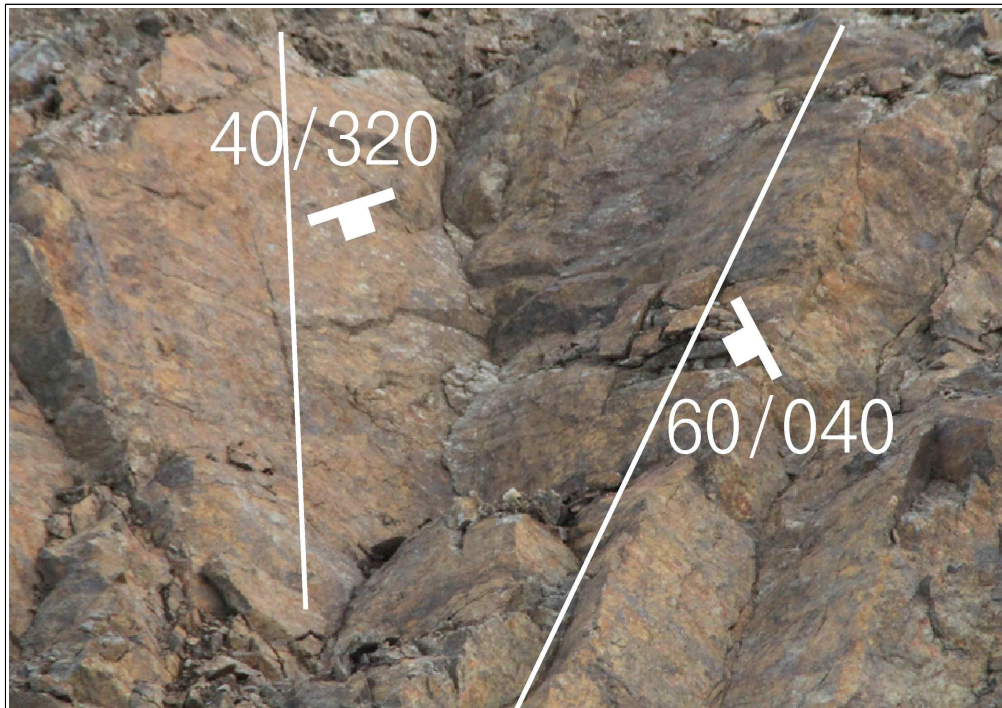
【그림 19】 B 영역에 발달한 불연속면
