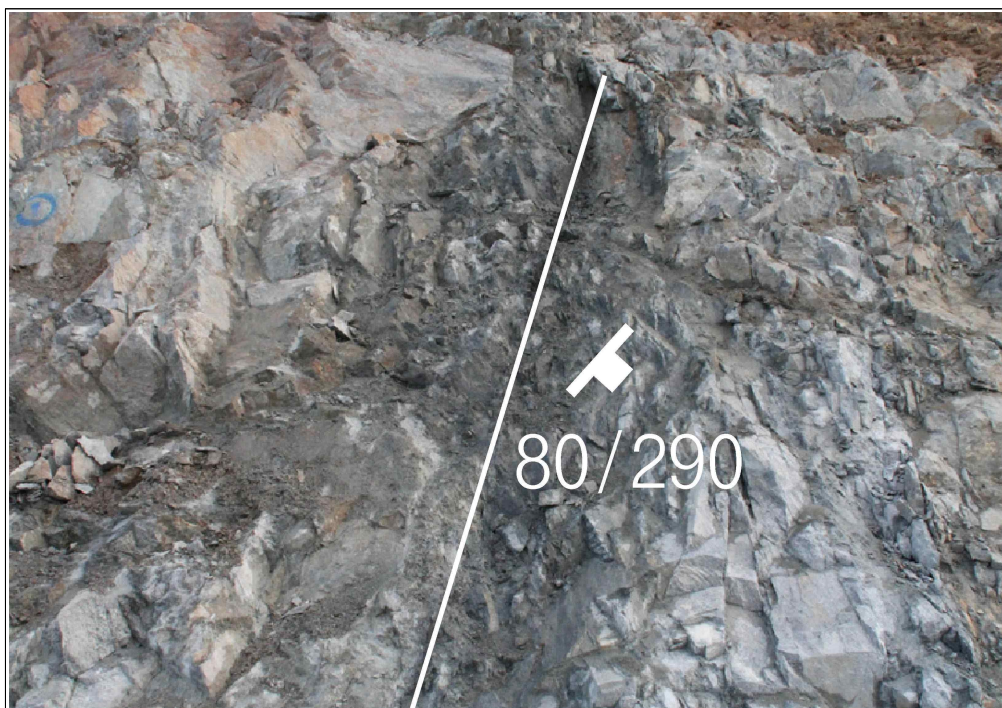
【그림 25】 C 영역에 발달한 불연속면
