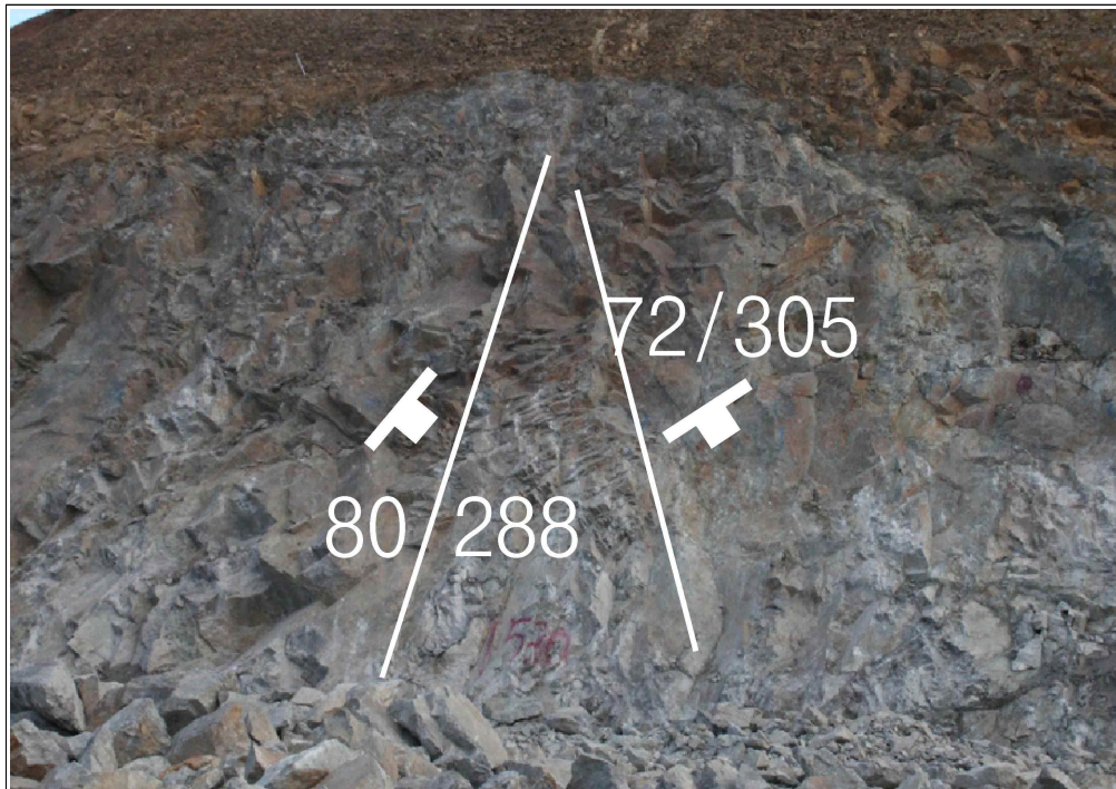
【그림 14】 A 영역에 발달한 불연속면
