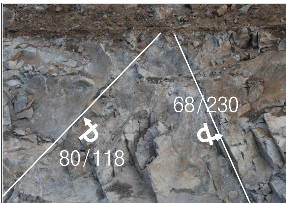
【그림 27】 C 영역에 발달한 불연속면
