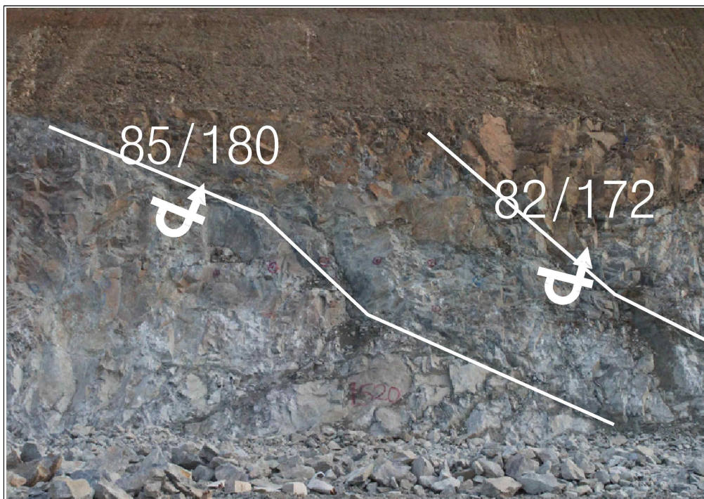
【그림 16】 B 영역에 발달한 불연속면
