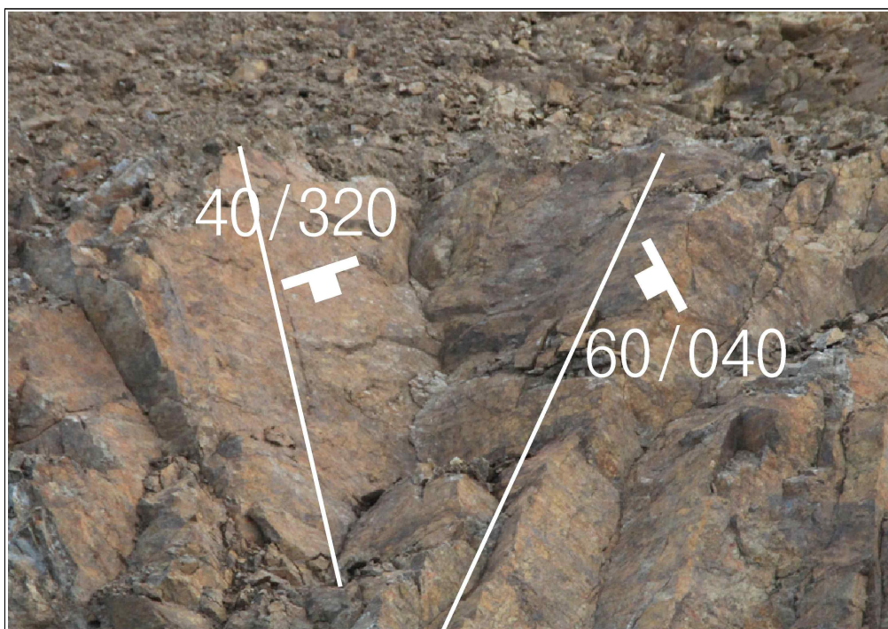
【그림 18】 B 영역에 발달한 불연속면
