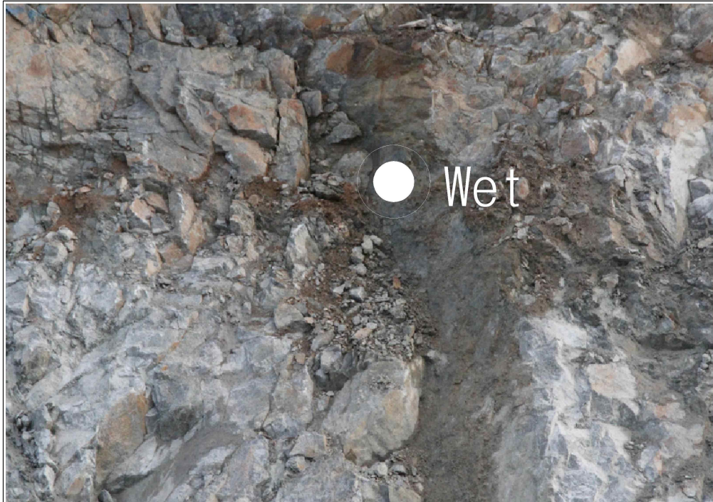
【그림 21】 B 영역 상세사진 (지하수 유출)
