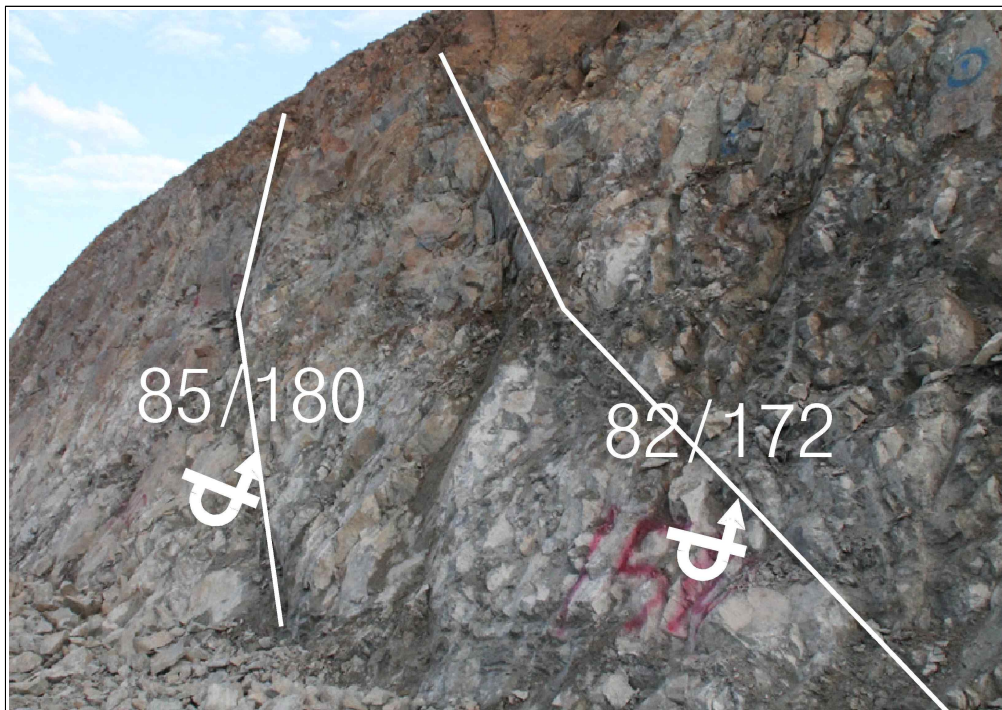
【그림 17】 B 영역에 발달한 불연속면
