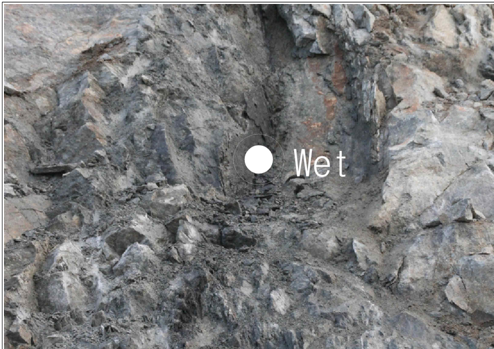
【그림 28】 C 영역 상세사진 (지하수 유출)
