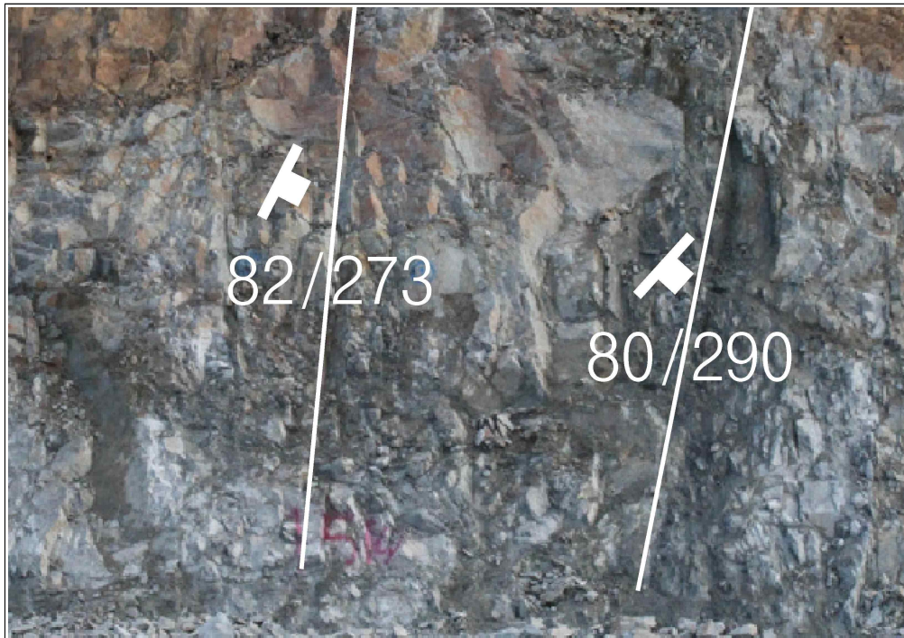
【그림 24】 C 영역에 발달한 불연속면
